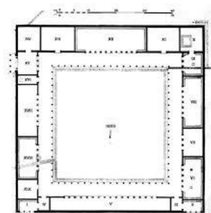
Фиг. 8 План на гимназион с екседри, отворени към портика
