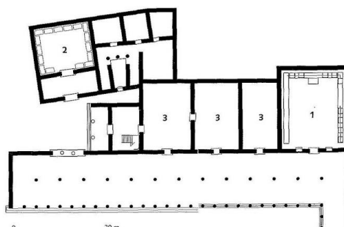
Фиг. 7 а Библиотеката на Пергамон : 1 – библиотечна зала с шкафове за книги, използвана като читалня и Пергамска школа
